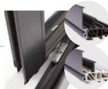
FINITION INTÉRIEURE DU DORMANT ADAPTÉE AU CHOIX D'AMBIANCE
