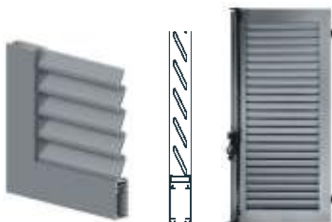
À la française
