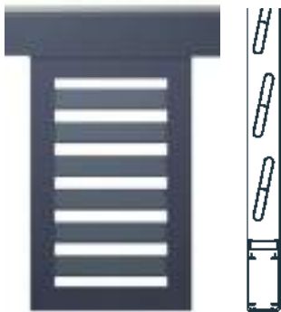
Lames inclinées 68 x 10 mm
