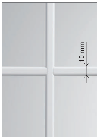
Petits bois ALU TRADI Blanc Section 10x8 mm
