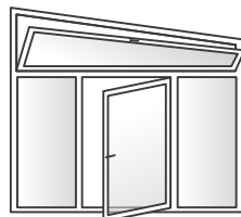
CHÂSSIS JUXTAPOSÉ AVEC FRAPPES
