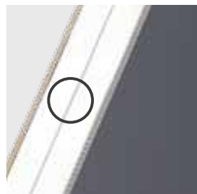
TÔLE ALUMINIUM EN OPTION POUR PLUS DE SÉCURITÉ TÔLE ALUMINIUM DE 1,8 mm D'ÉPAISSEUR POUR AMÉLIORER LA SÉCURITÉ SUR TOUS LES MODÈLES Y COMPRIS LES MODÈLES VITRÉS
